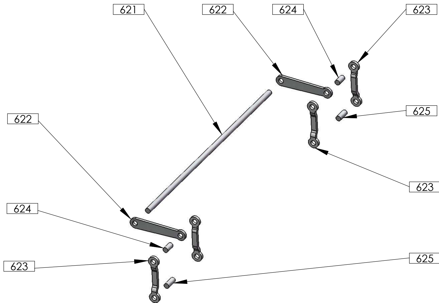
Détail bielle de renvoi 623
