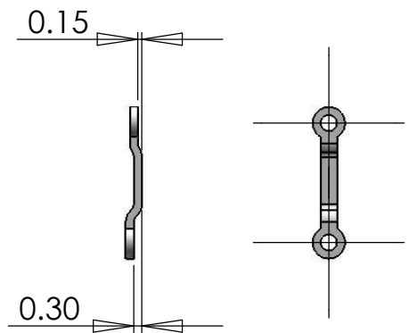
Détail bielle de renvoi 623
